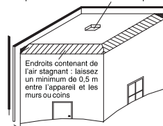
a) Fixation au plafond
